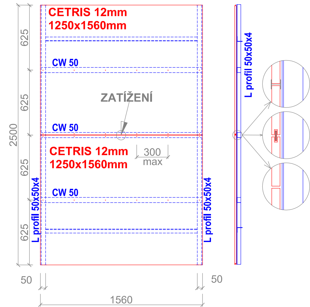
Vzorek 3 - CETRIS Basic 12 mm 3 příčné výztuhy profily CW 50
