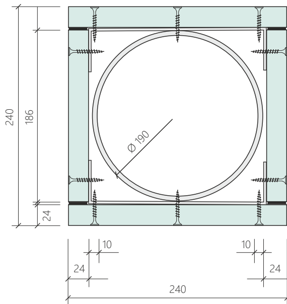
a) obklad kruhových uzavřených profilů
